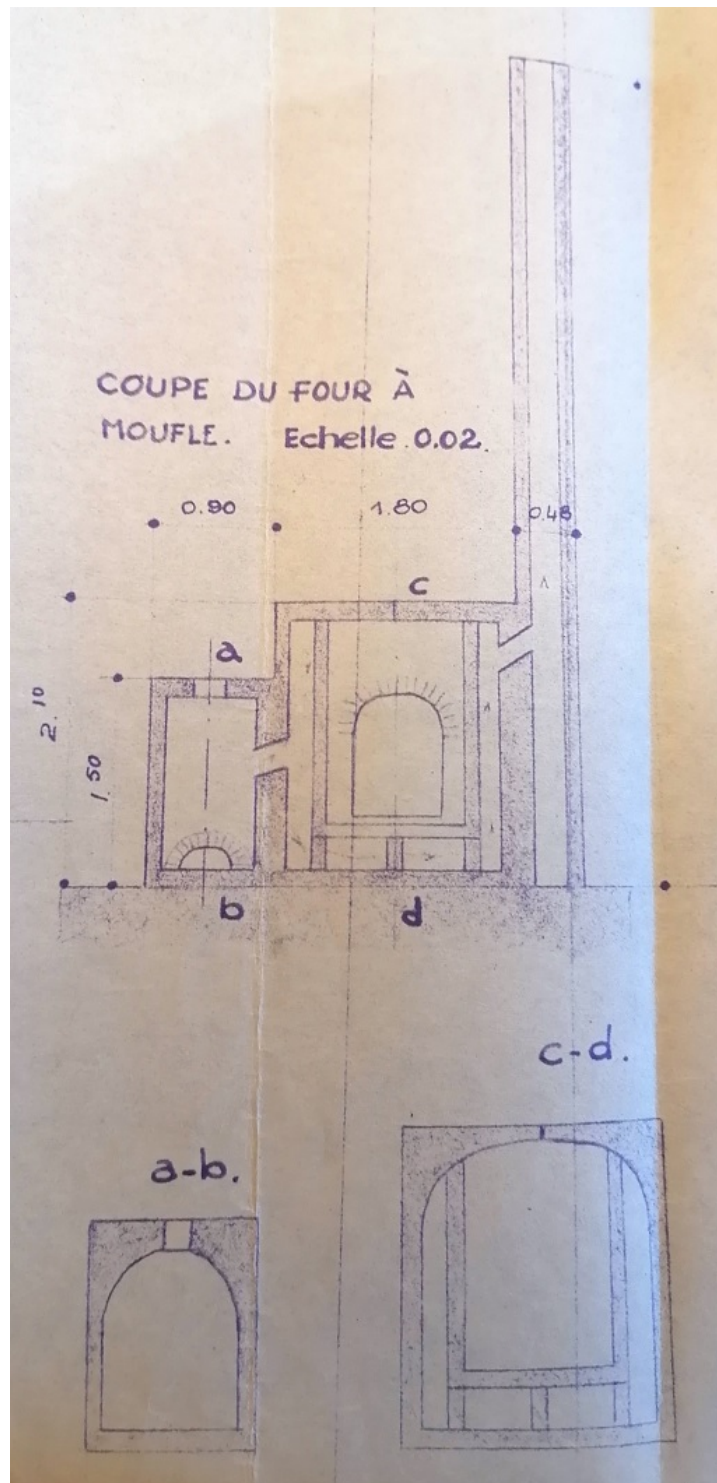
Figure 4 - coupes du four de la famille LAMY - dessin de 1945 (A.D.14)
